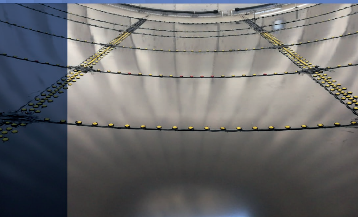
Tanques de aço parafusados revestimento vitrificado
